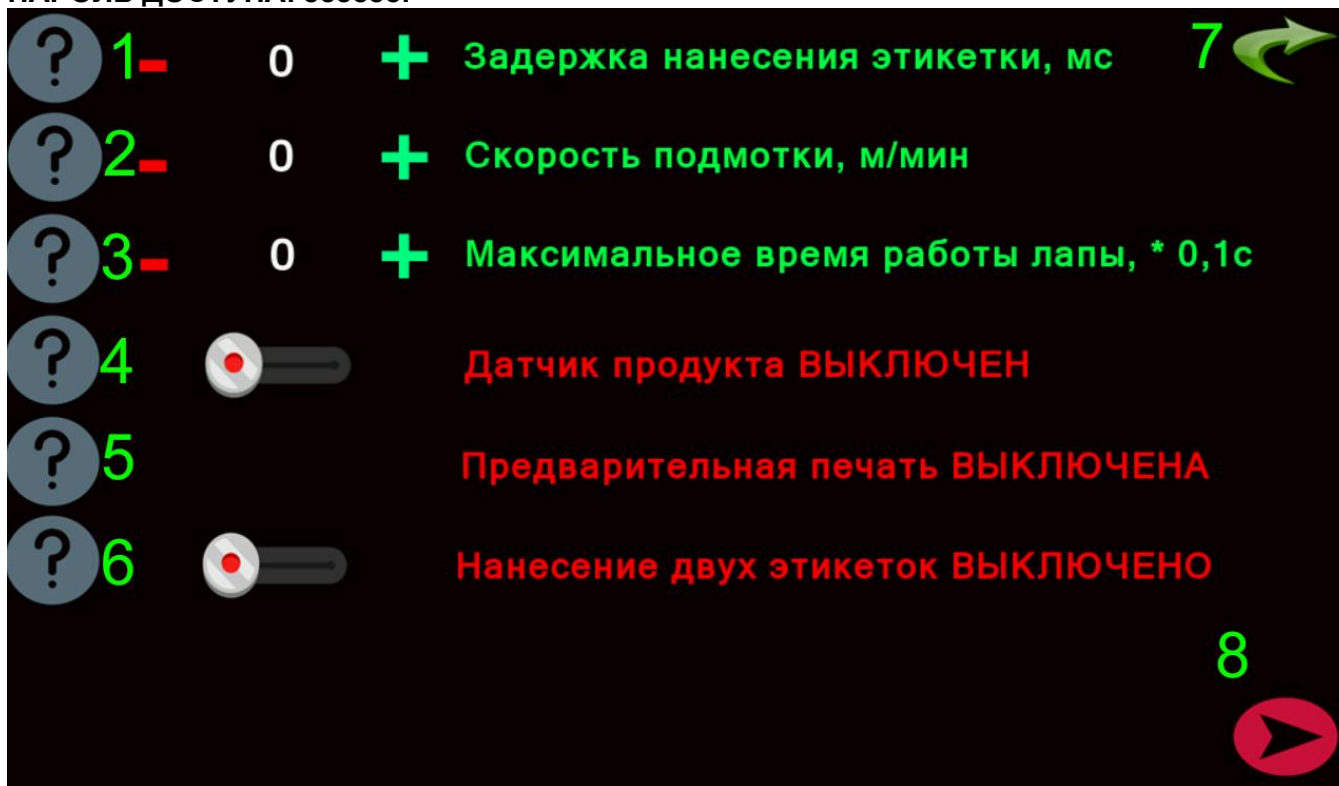
Рисунок 2.11. Меню основных настроек.
