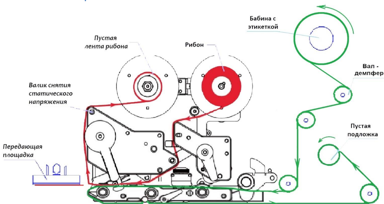
Рисунок 2.2. Схема заправки принтера-аппликатора Н-ПР-03Д.
