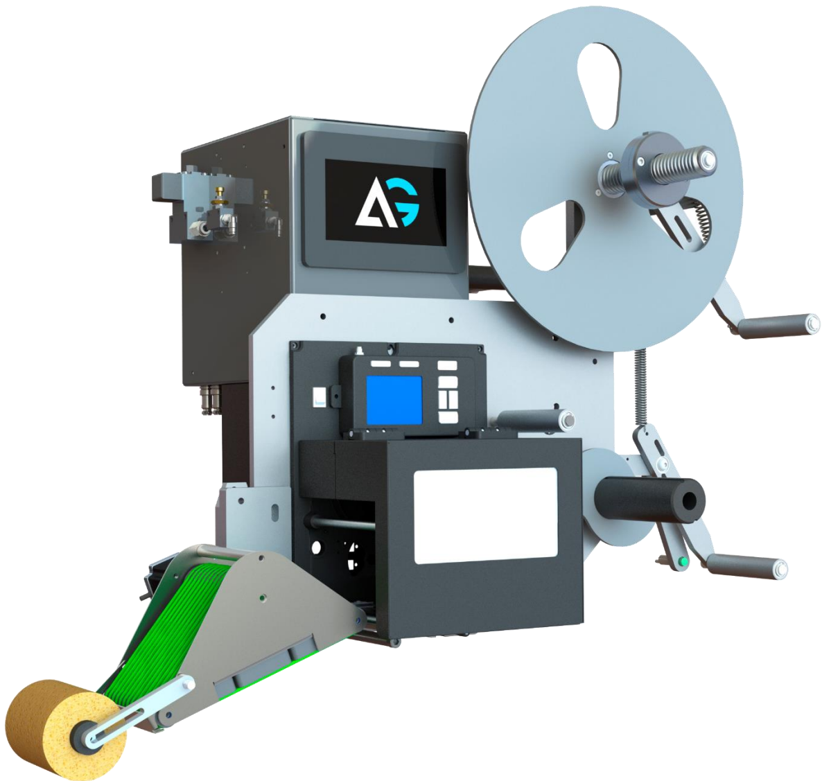
Рисунок 2.2. Общий вид принтера-аппликатора Н-ПР-04 без стойки.
