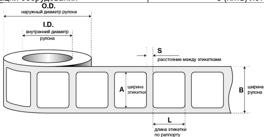
Рисунок 1.3. Характеристики этикетки для Принтера-аппликатора Н-ПР-04
