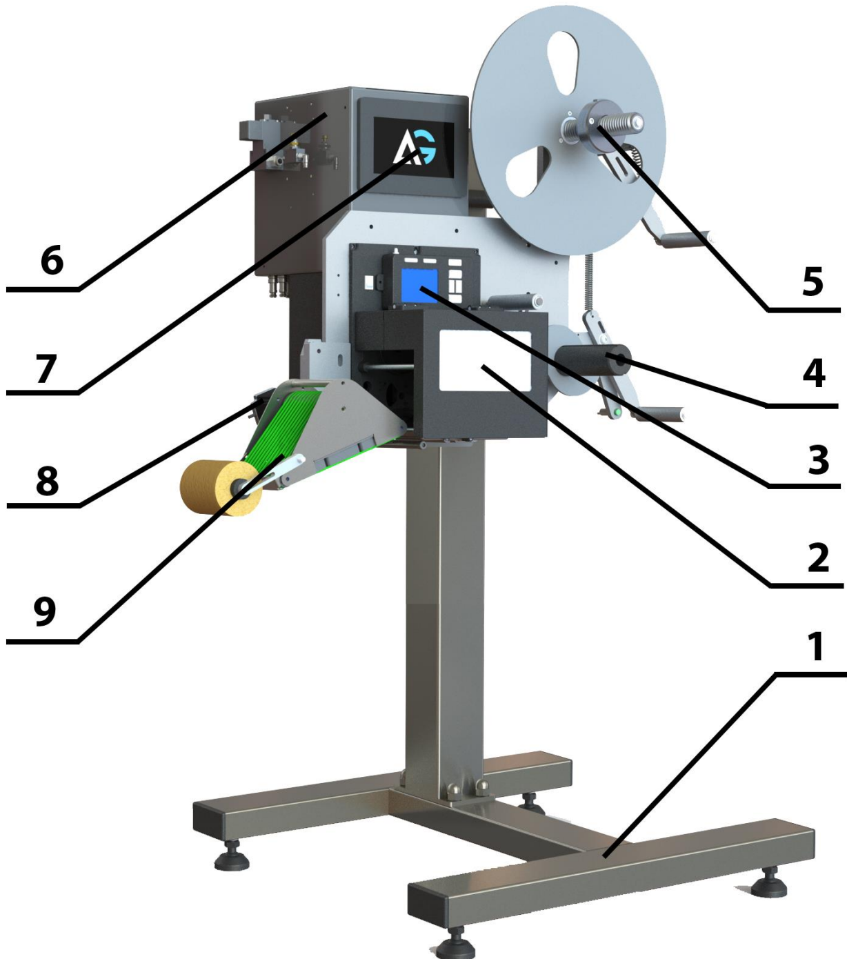
Рисунок 2.1. Внешний вид установки Принтера-аппликатора Н-ПР-04.
