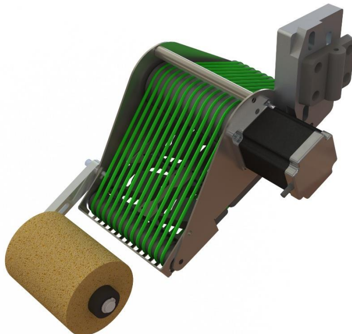
Рисунок 1.4. Модуль переноса этикетки принтера-аппликатора Н-ПР-04.
