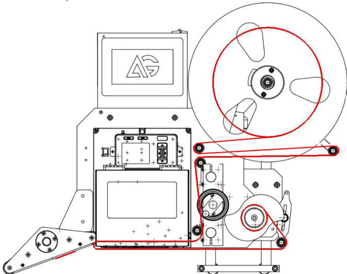
Рисунок 3.1. Схема заправки принтера-аппликатора Н-ПР-04.
